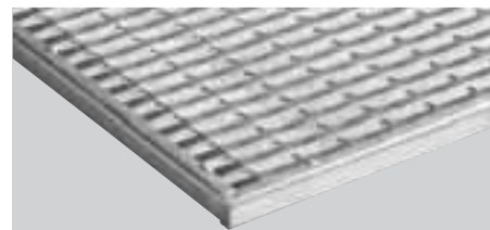
Grigliato in acciaio zincato a maglie, maglie 9 x 31 mm
